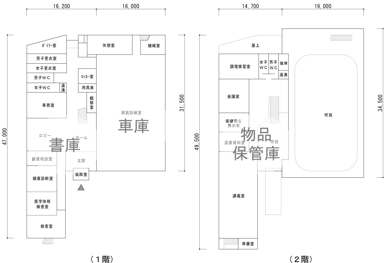
福光保健センター現況平面図
