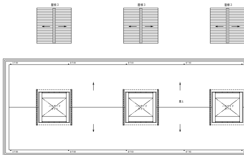
体育館 キョウトワークレベル 平面図
