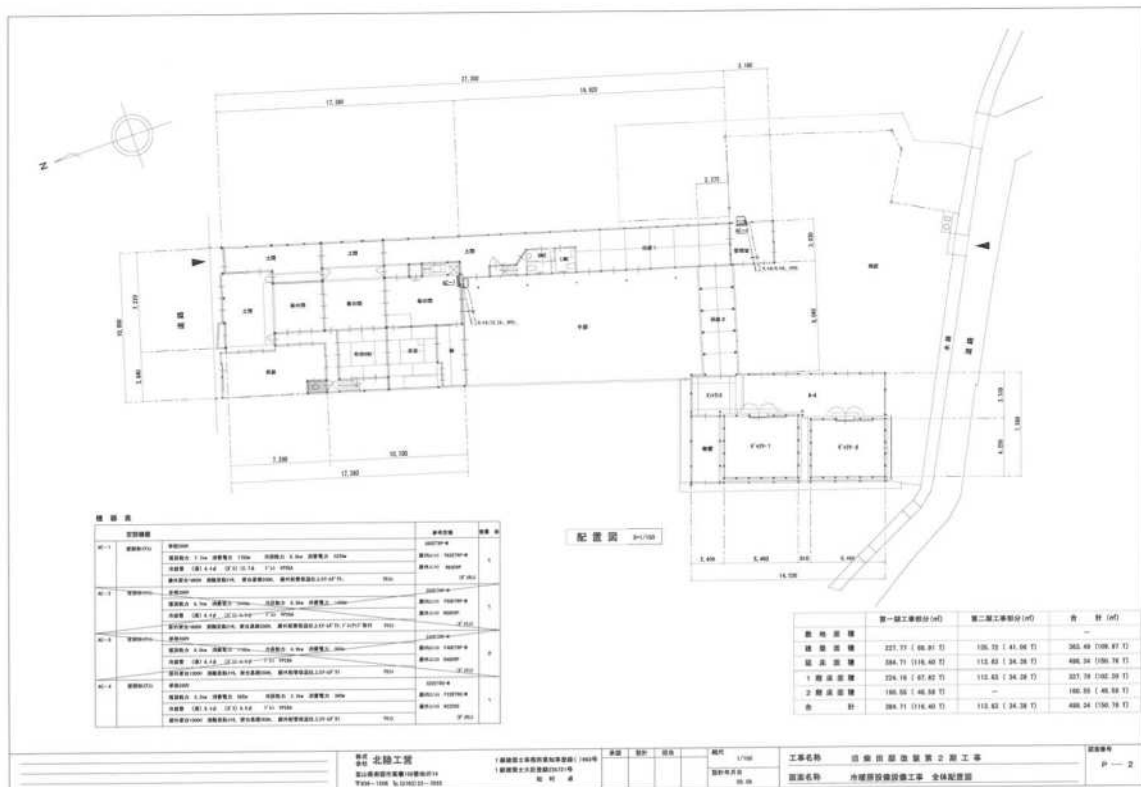
配置図
