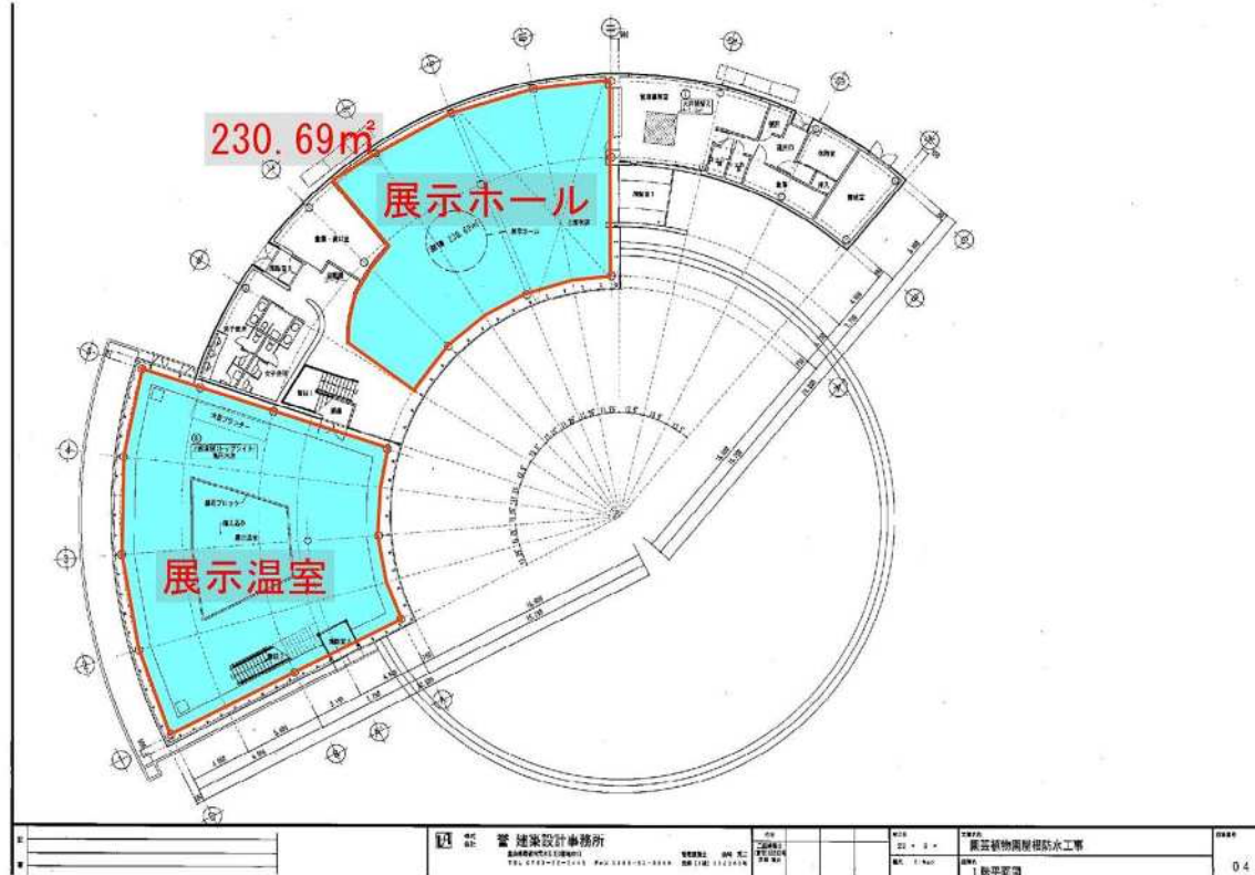
平面図（1階）
