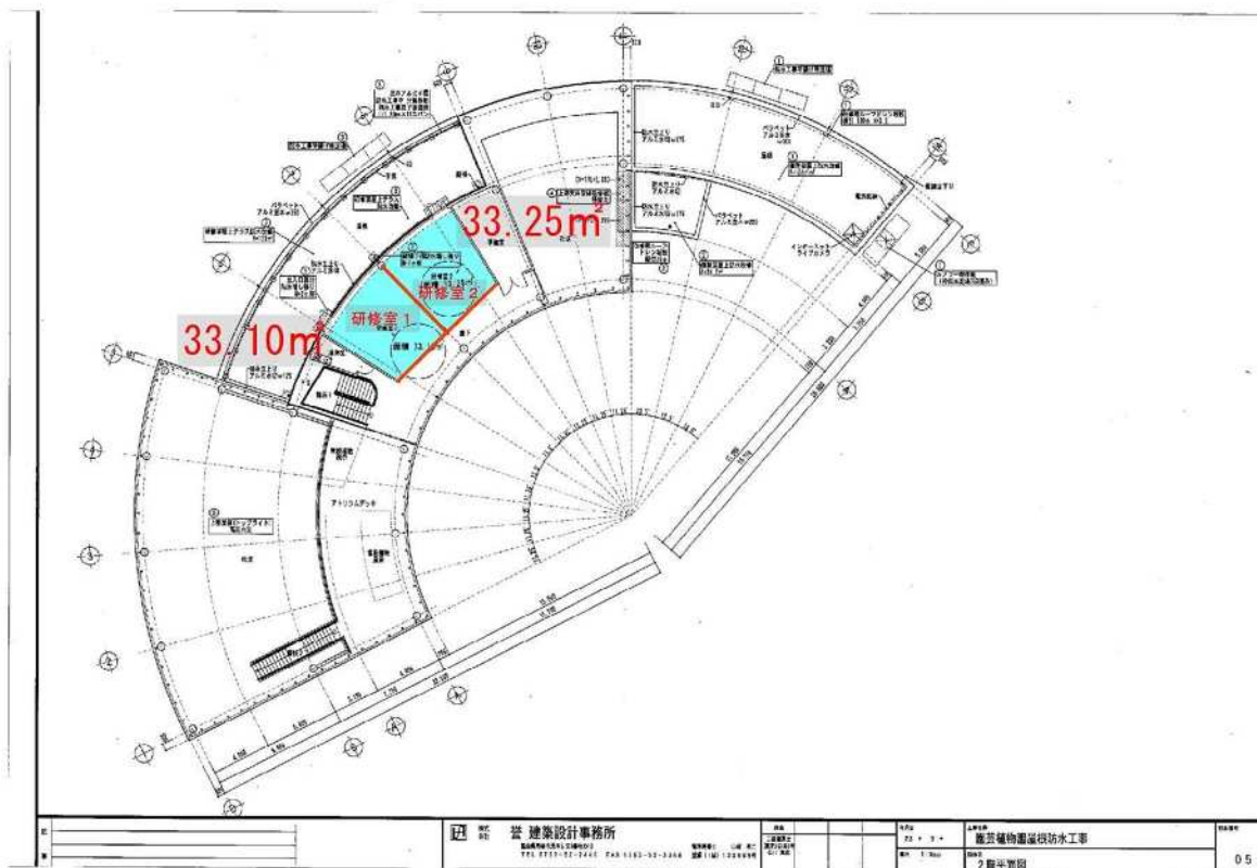
平面図（2階）
