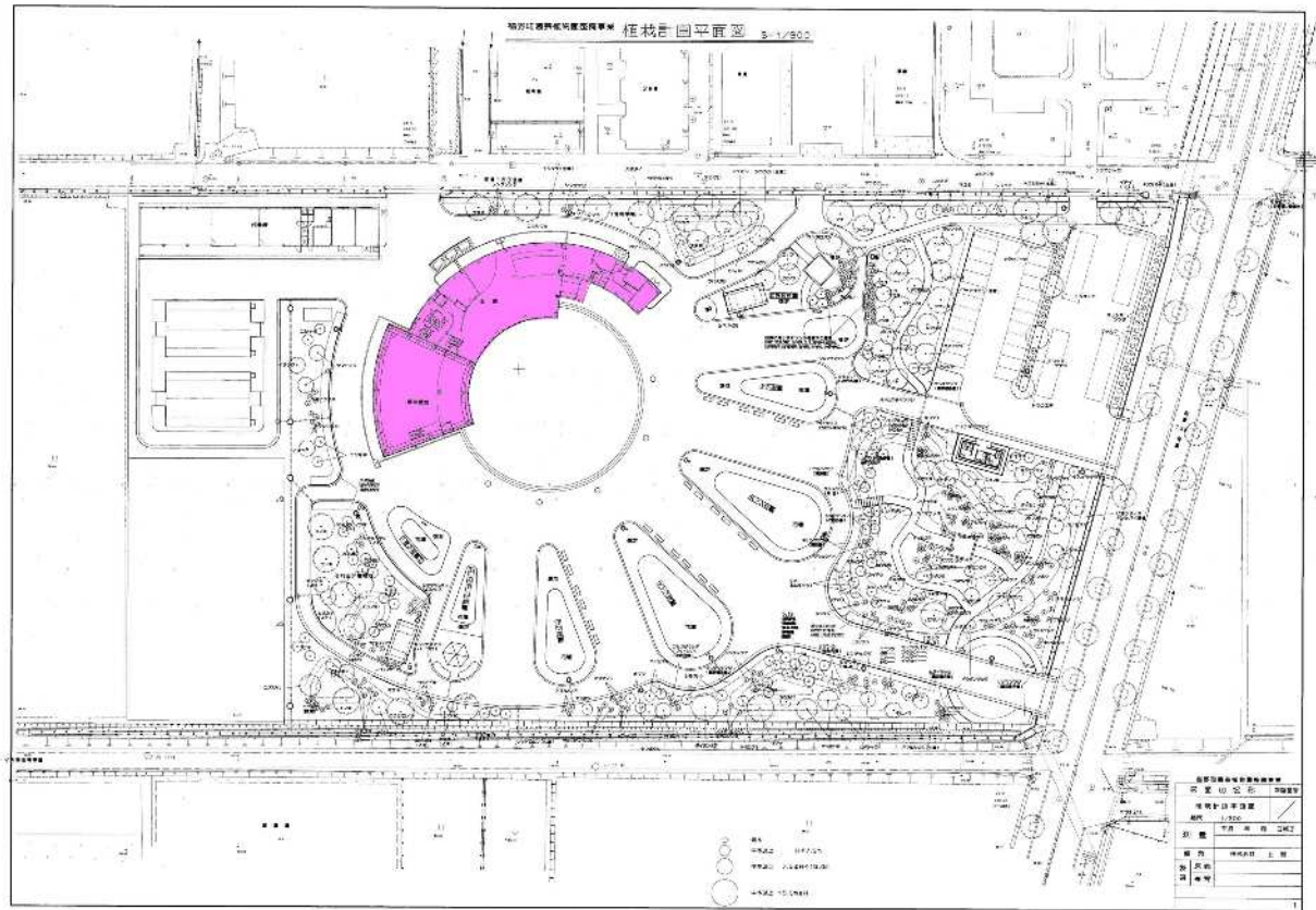
植栽図
