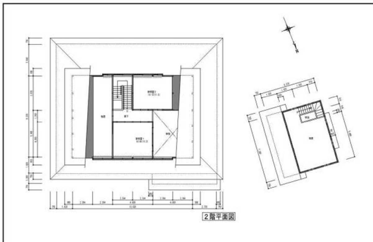
2階平面図
