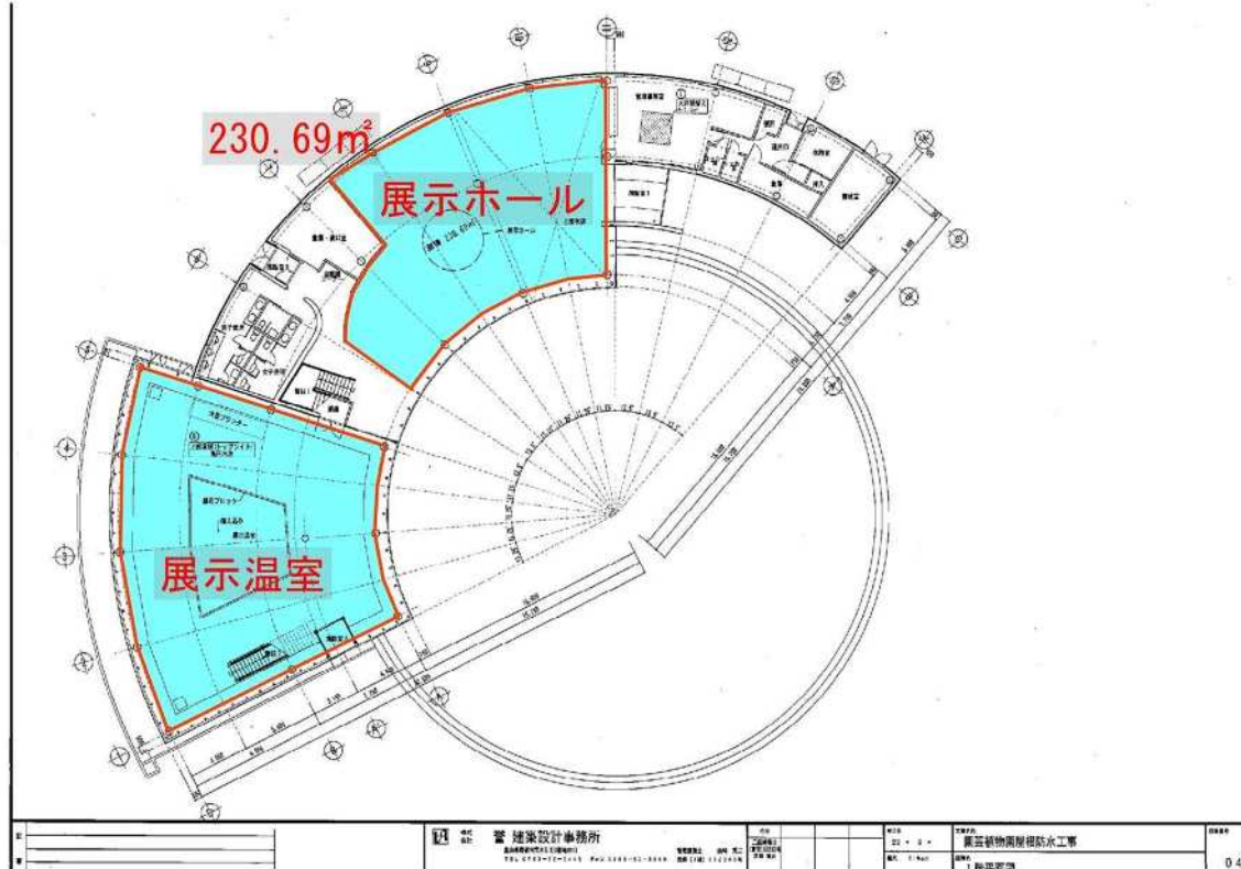
平面図 (1階)
